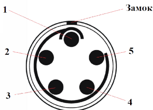
Распиновка порта LEMO (5-pin) приемника AlphaGEO A8:
